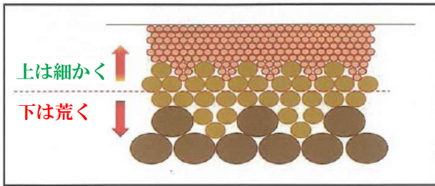
団粒構造モデル
